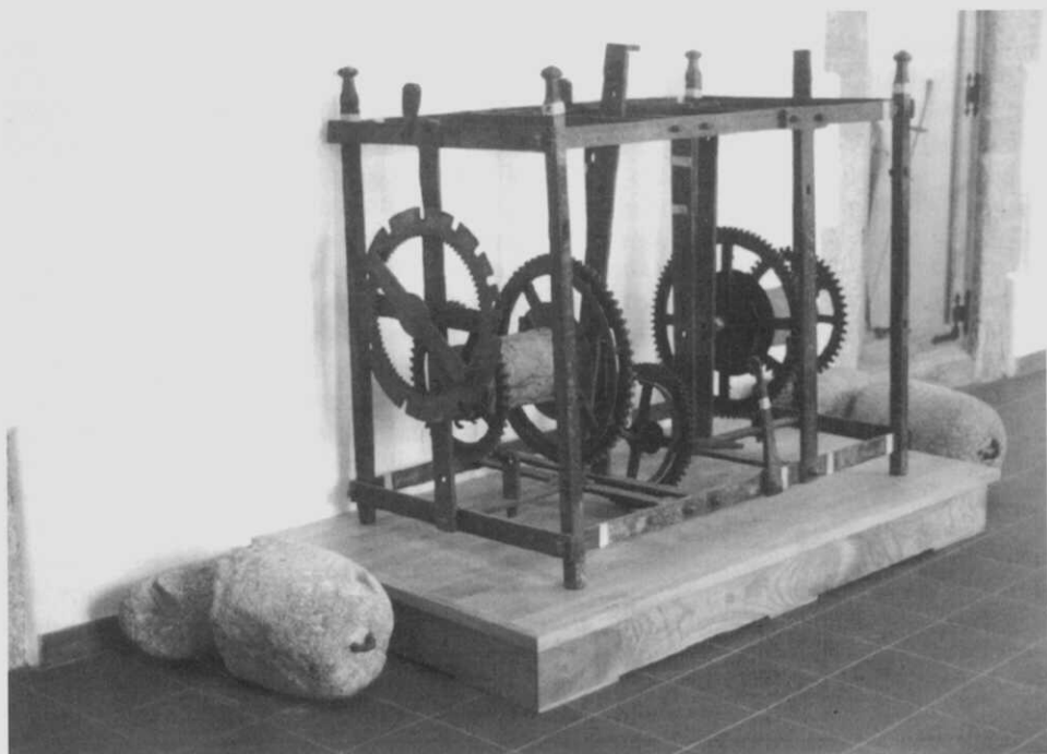
Fig. 2.- Maquinaria do reloxo, construído por Lombardero no 1757 e hoxe conservado no Museo das Mariñas.
